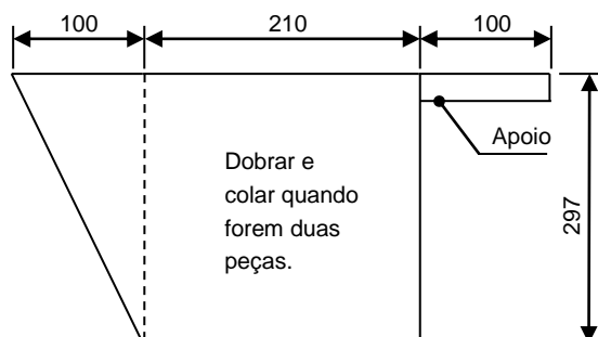
Figura A.1 (b) – Molde para dispositivo – Dimensões em mm
