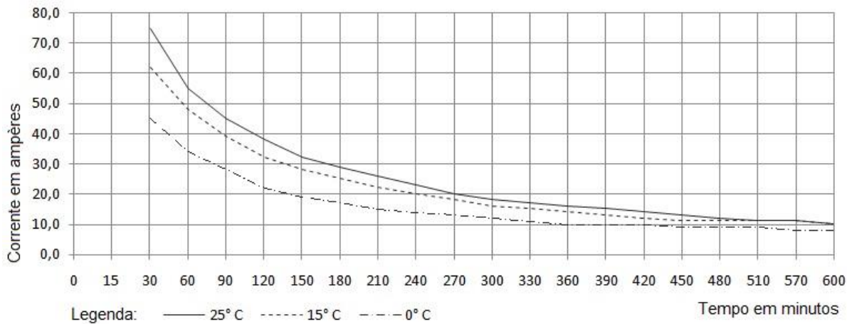
Figura B.3 – Exemplo de rendimento de uma bateria em diferentes temperaturas em função do tempo de descarga
